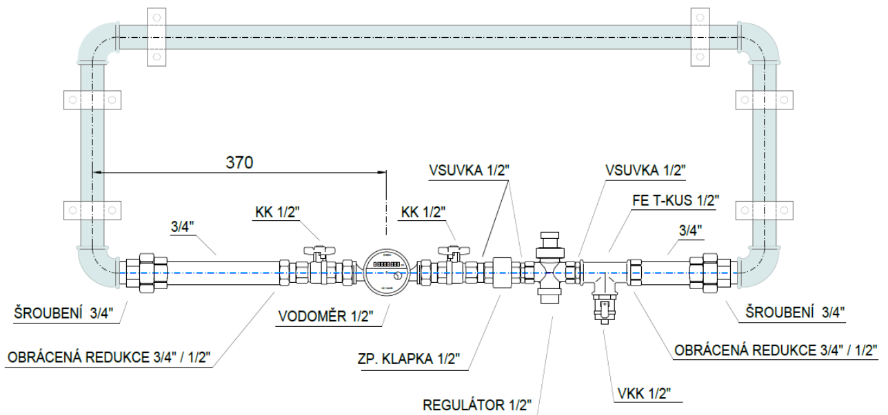
SESTAVA VODOMĚRU
