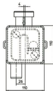
Podomítková vodní a mechanická zápachová uzávěrka HL138
