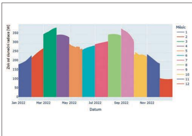
Obr. 4. Příklad výstupu – graf simulovaných hodnot tepelných zisků fasády od sluneční radiace v průběhu roku – software FSVM.
