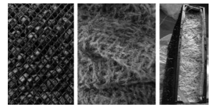
Obr. 4 – Ukázka zkoušených materiálů zprava - keramzit, kokosová rohož a dřevovlna.
